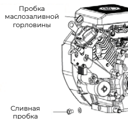
Рис. 3. Проверка уровня моторного масла
